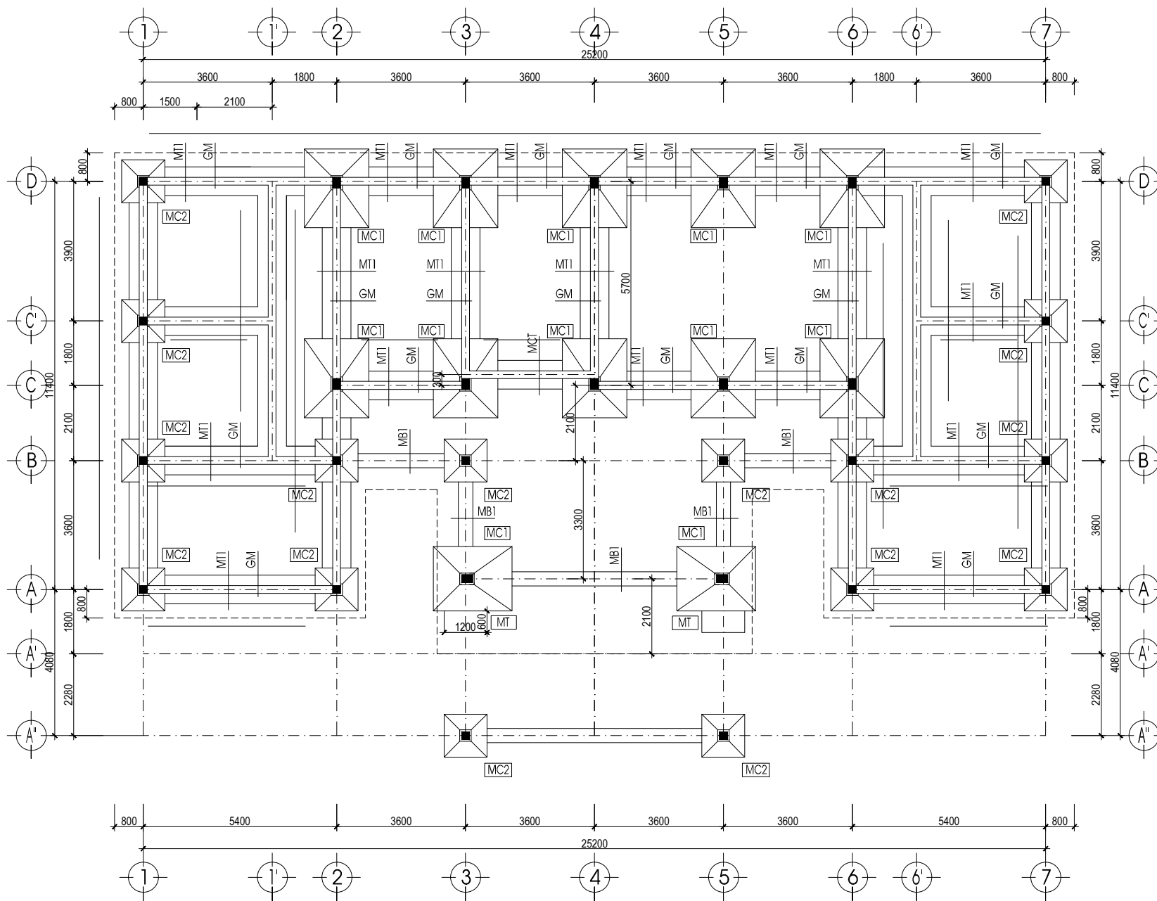
MẶT BẰNG MÓNG
